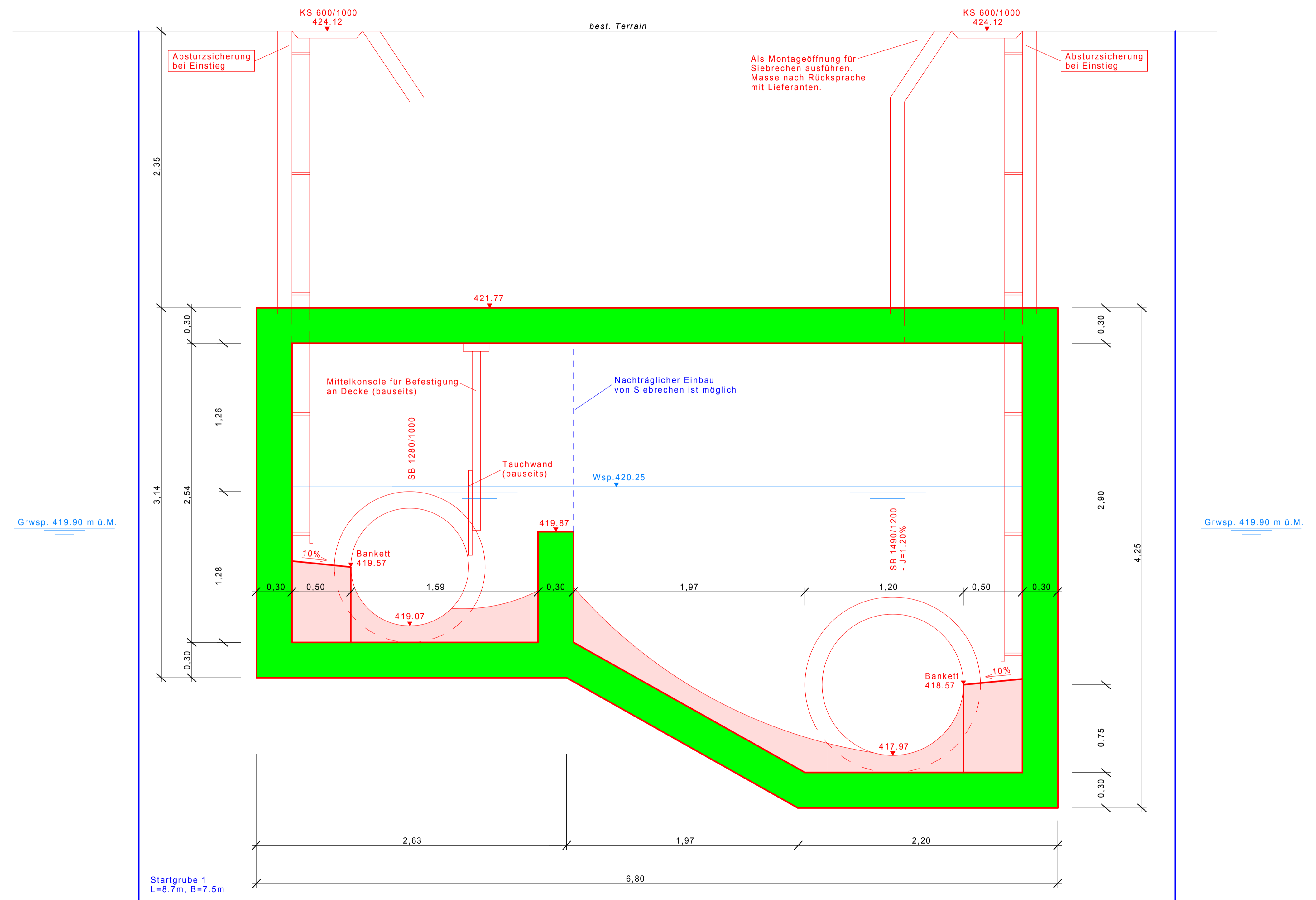
Schnitt A-A 1:20
